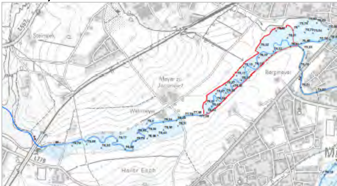
Karte 9: Fünfjähriges Hochwasser im Bereich der östlichen Johannisbachaue
